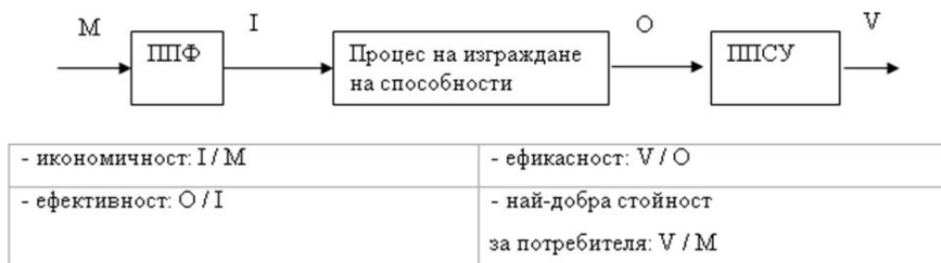
Фиг. 2. Връзка „икономичност – ефективност – ефикасност – най-добра стойност за потребителя“
